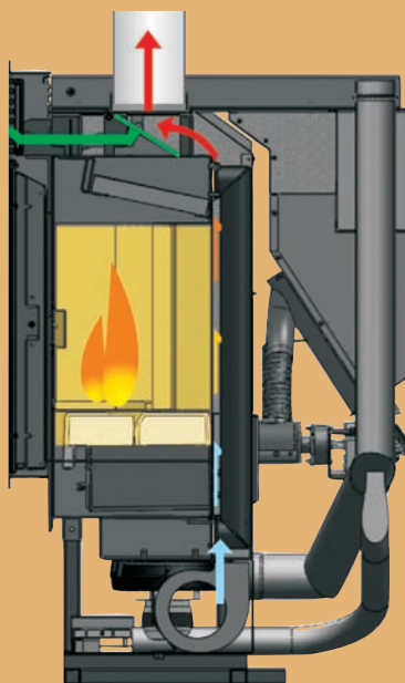
Teplý vzduch vháněný do rozvodů
