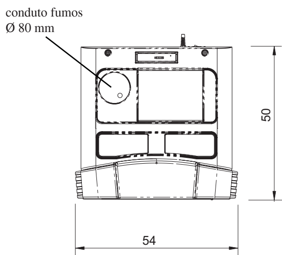
PLANTA
