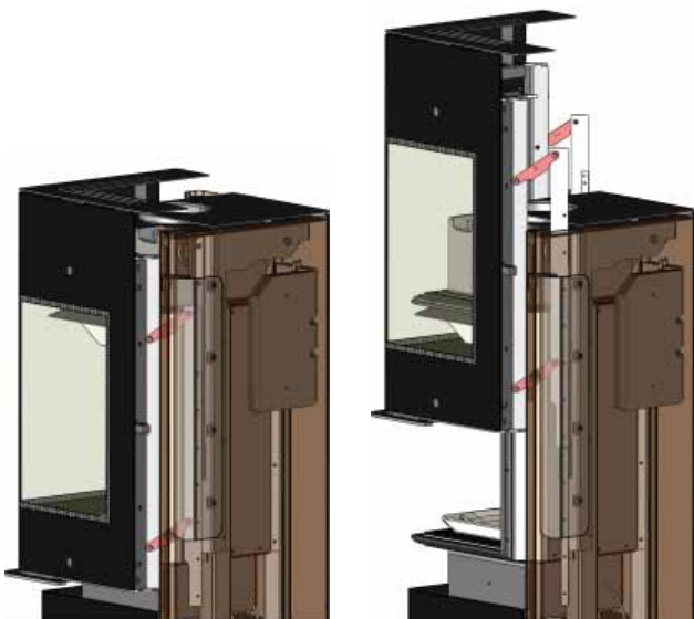
Abb. 3 - Spezielle Schiebetür
